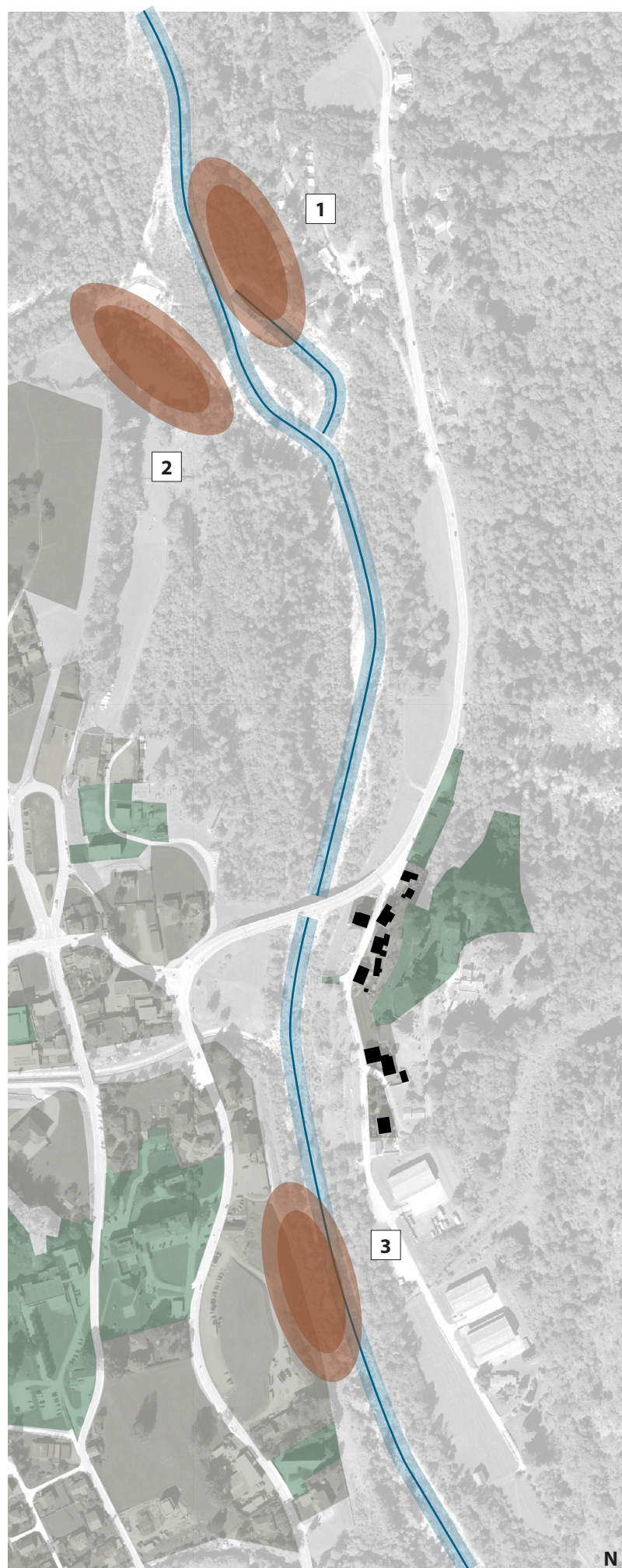
Il fiume Brenno - concetto di riqualifica e accessibilità - Scala 1:5'000
