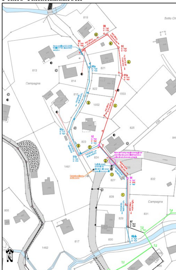
Piano canalizzazioni
