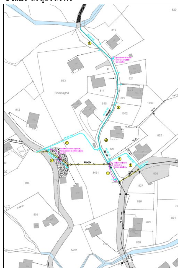
Piano acquedotto
